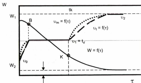
Hình 8.4. Sự biến đổi độ ẩm và nhiệt độ của vật liệu theo thời gian sấy
