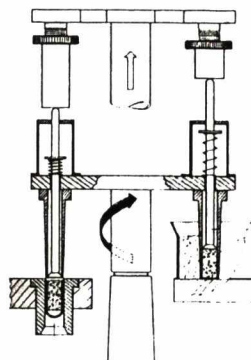
Hình 12.12. Chuyển động của vít phân liệu
