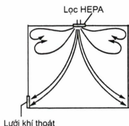
Hình 13.3. Mô hình thổi khí không theo một chiều
