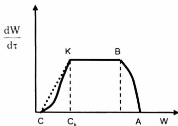
Hình 8.6. Đường cong tốc độ sấy
