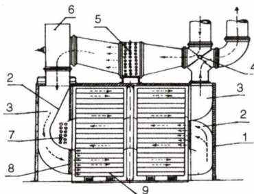
Hình 8.7. Nguyên tắc cấu tạo phòng sấy
