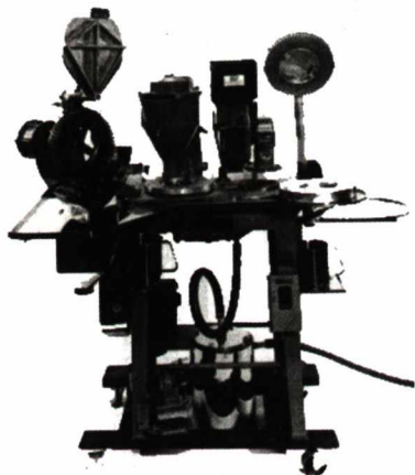
Hình 12.8. Máy đóng nang bán tự động
