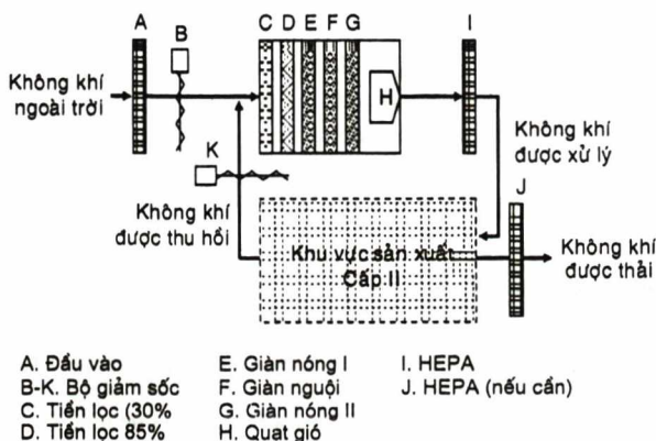
Hệ thống xử lý không khí với lọc HEPA
