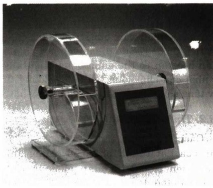
Hình 9.10. Máy đo độ mài mòn, hiệu ERWEKA
