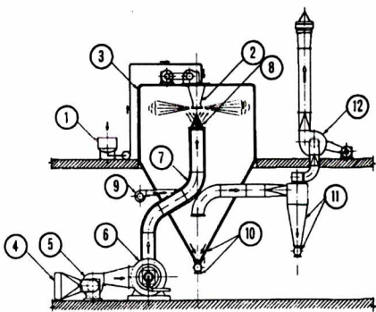
Hình 8.13. Sơ đồ máy sấy phun
