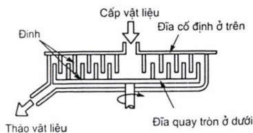
Hình 6.3. Máy xay đinh
