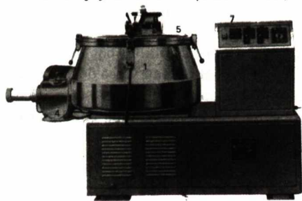
Hình 10.21. Máy tạo hạt cao tốc
