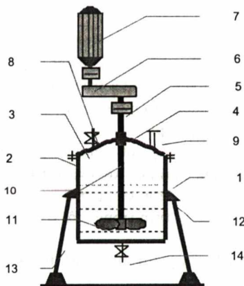
Hình 7.1. Sơ đồ cấu tạo thiết bị khuấy
