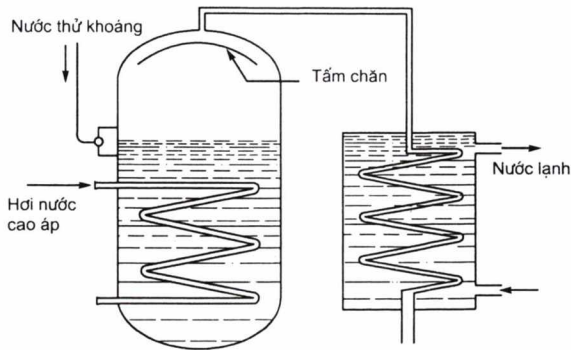
Hình 13.9. Sơ đồ máy cất nước
