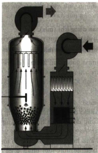
Hình 8.10. Sơ đồ máy sấy tầng sôi
