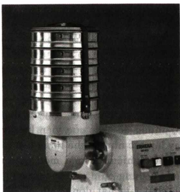
Hình 9.9. Thiết bị phân loại cỡ hạt, hiệu ERWEKA
