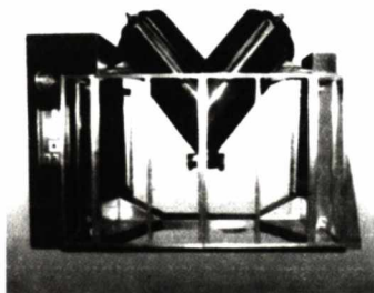
Hình 7.9. Các loại thùng trộn a) Thùng trộn hai đầu hình côn; b) Thùng trộn chữ V.
