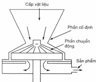
Hình 6.6. Máy xay kéo
