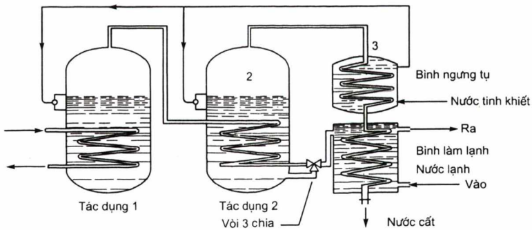
Hình 13.10. Máy cất nước có tác động kép
