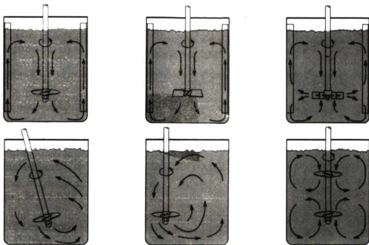
Hình 7.5. Các kiểu đặt cánh khuấy
