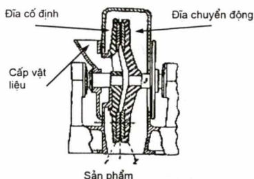
Hình 6.4. Máy xay đĩa
