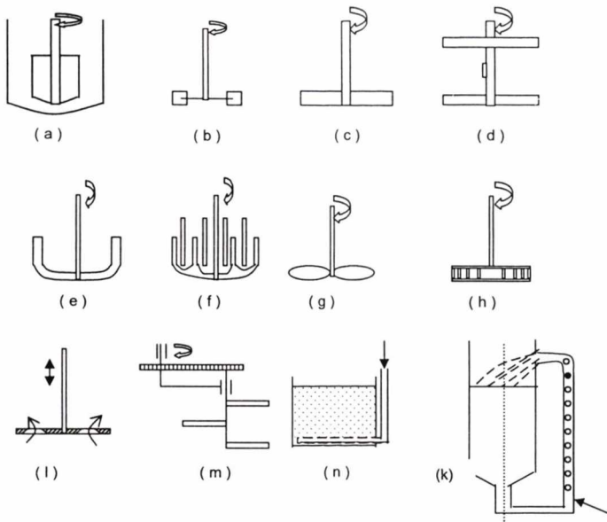
Hình 7.2. Các loại cánh khuấy:
