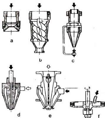
Hình 8.12. Các loại vòi phun
