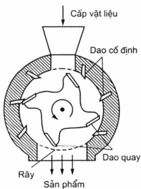
Hình 6.2. Máy xay cắt
