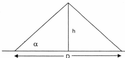
Hình 9.2. Đo góc nghỉ \alpha của khối bột hình nón
