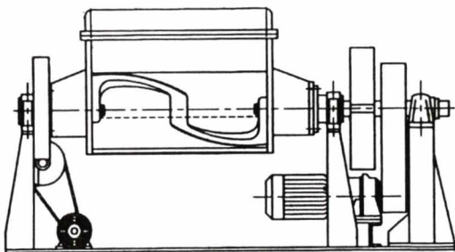
Hình 7.7. Sơ đồ thiết bị nhào trộn
