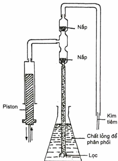
Hình 13.11. Nguyên tắc đóng từng ống
