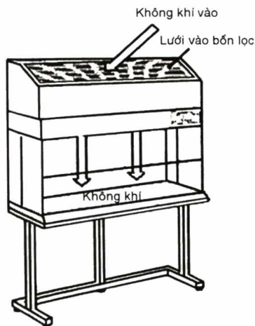
Hình 13.6. Buồng thổi khí song song một hướng theo phương thẳng đứng
