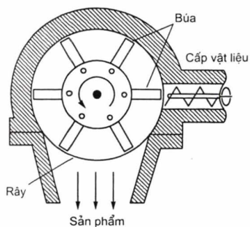
Hình 6.1. Máy xay búa
