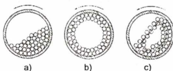
Hình 6.5. Máy nghiền bi
