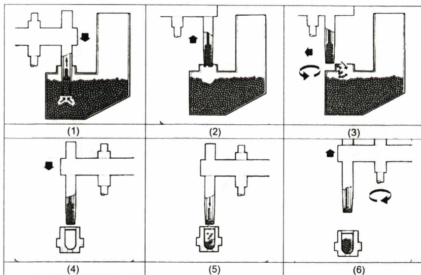
Hình 12.13. Nguyên lý đóng vi hạt vào nang của vít phân liệu
