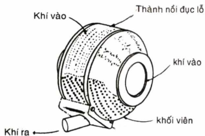
Hình 11.3. Thiết kế của nồi bao đục lỗ
