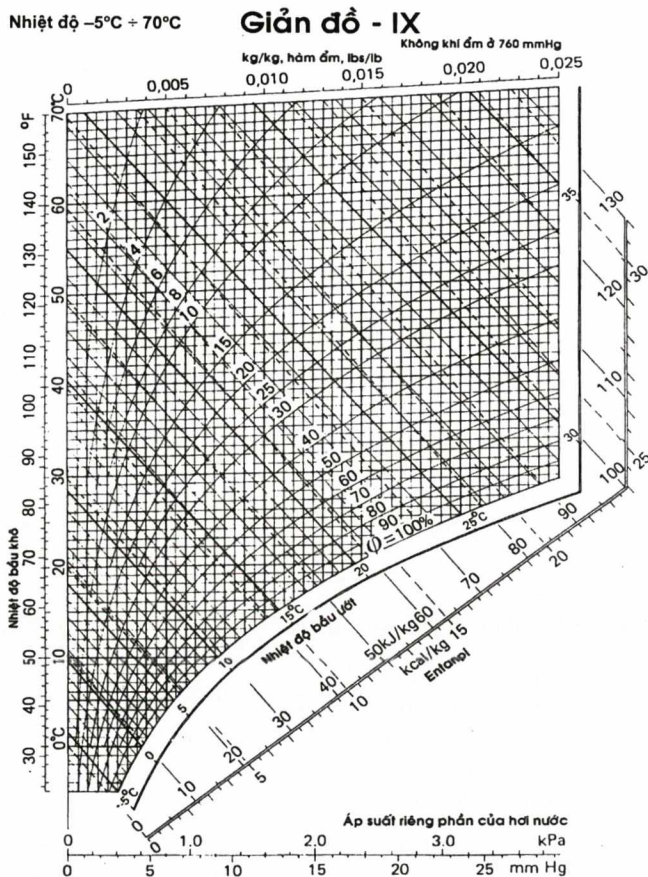
Hình 8.2. Giản đồ không khí ẩm
