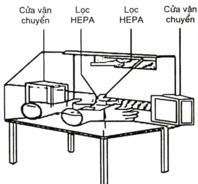
Hình 13.7. Buồng cô lập, sạch, có xử lý không khí ra
