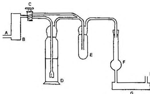
Hình 1: Thiết bị tạo hơi thủy ngân
