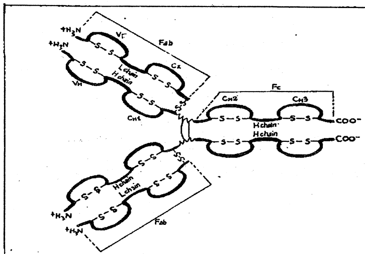
Hình 5.2: Cấu S-S, các domain và các mảnh phân tử Ig.
