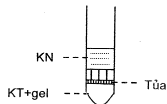
Hình 7.8. KN (lỏng) khuếch tán vào gel chứa KT, tại vị trí có nồng độ KN phù hợp sẽ tạo tủa, lắc không bị tan.
