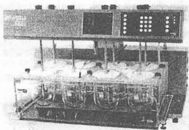
Hình 14.2. Máy đo độ hoà tan
