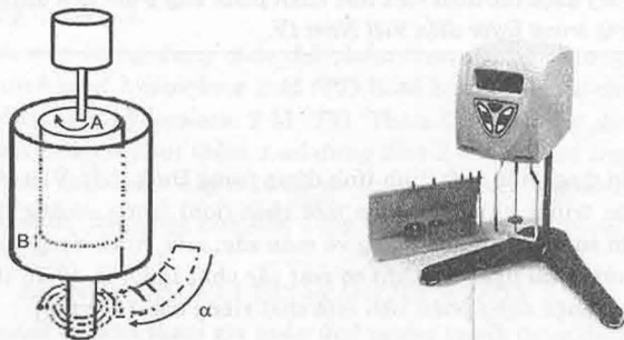
Hình 8.8. Nhớt kế quay
