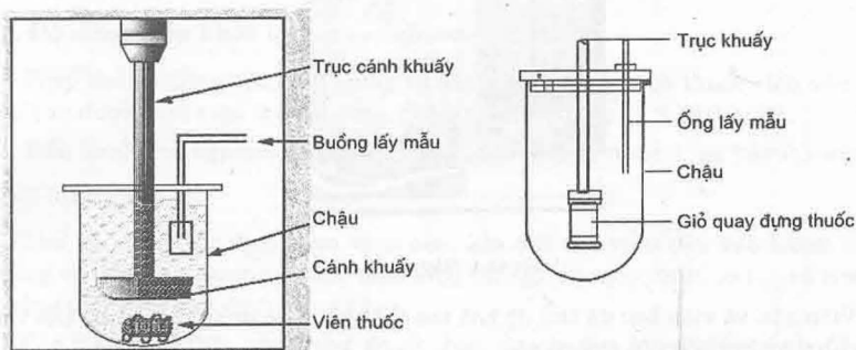
Hình 14.3. Cấu trúc của máy đo độ hoà tan
