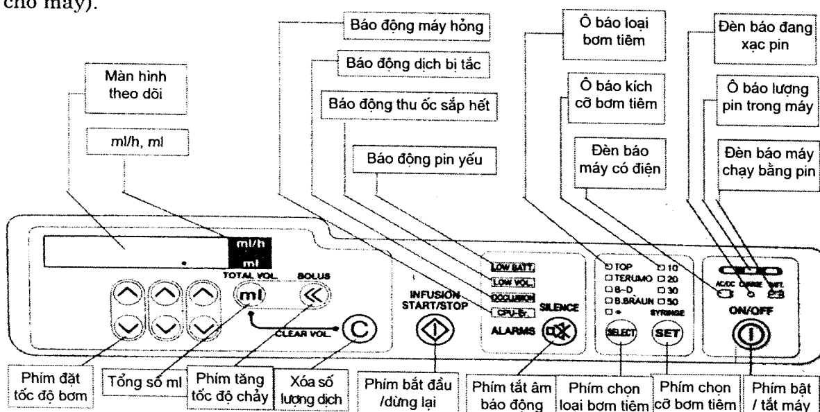
Hình 3. Bàn phím điều khiển của bơm tiêm điện
