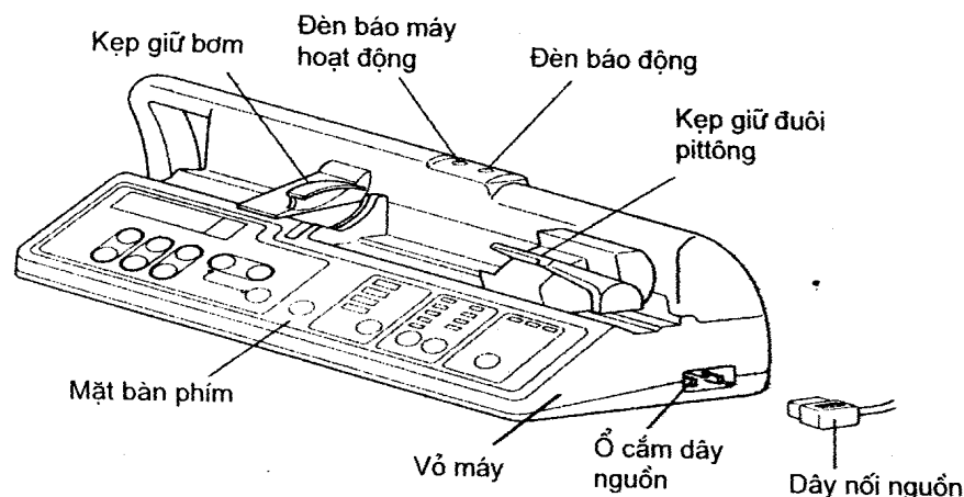
Hình 1. Mặt trước bơm tiêm điện
