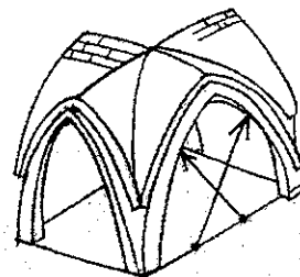
Mặt cắt và vòm mái có 2 tâm của kiến trúc Gôtích
