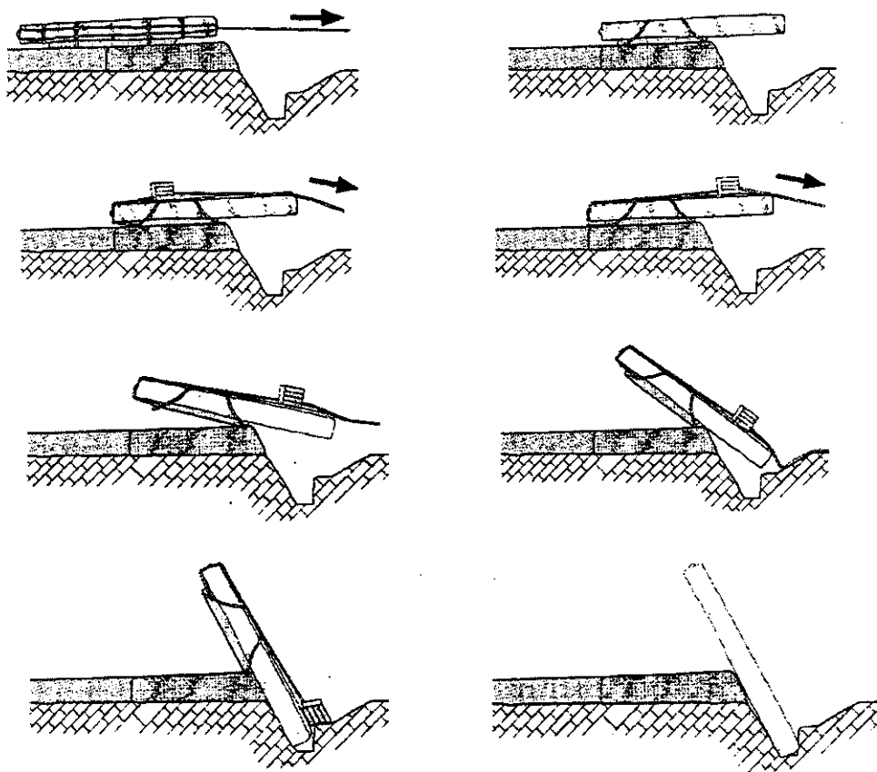
Các bước dựng phiến đá của cột đá
