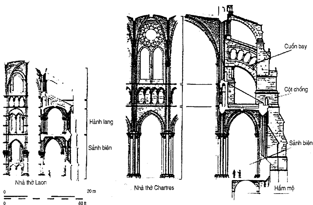
Một số bộ phận cấu tạo nhà thờ Gôtích
