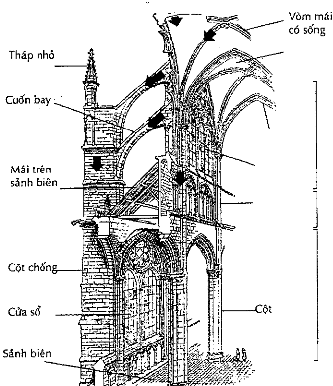
Hệ thống kết cấu Nhà thờ Gôtích
