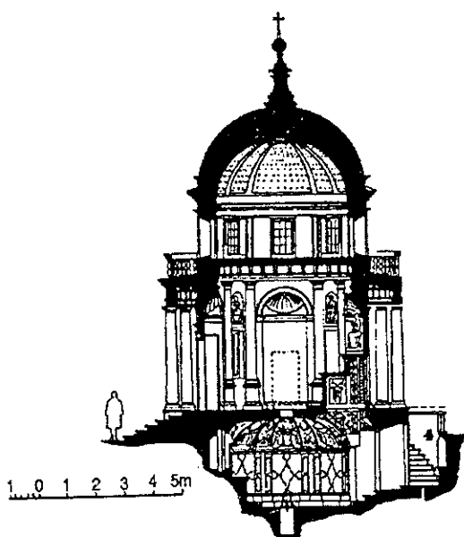
Mặt cắt đền Tempietto
