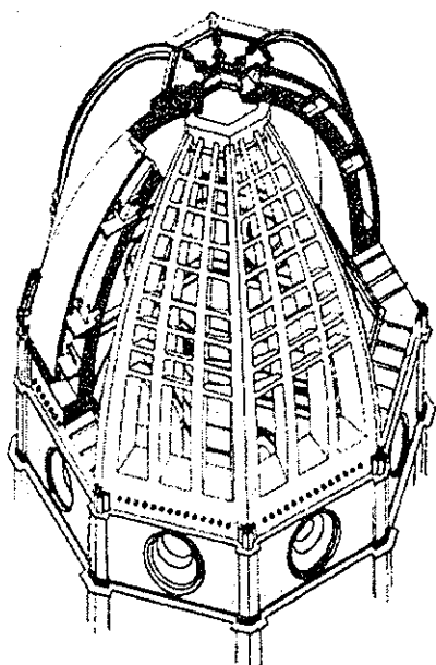
Mặt bằng, mặt cắt và cấu tạo vòm mái nhà thờ S. Maria del Fiore
