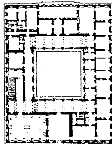
Mặt bằng lâu đài Farnese
