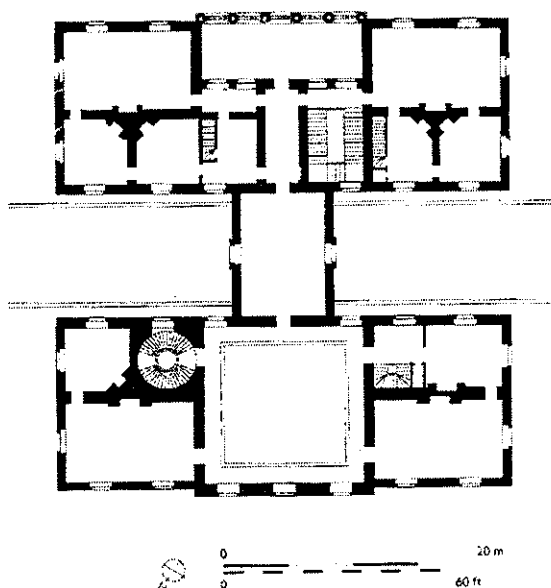
Mặt bằng Cung Nữ hoàng với đường chạy xe cút ngang tòa nhà ở điểm nút nối hai khối.
