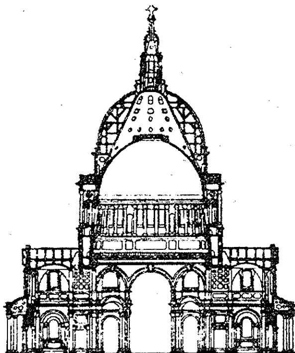
Mặt cắt nhà thờ St. Paul - London
