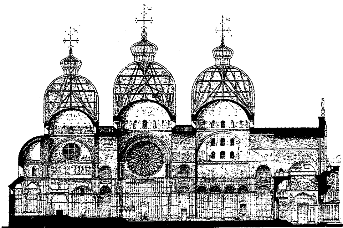
Mặt cắt nhà thờ S. Marco
