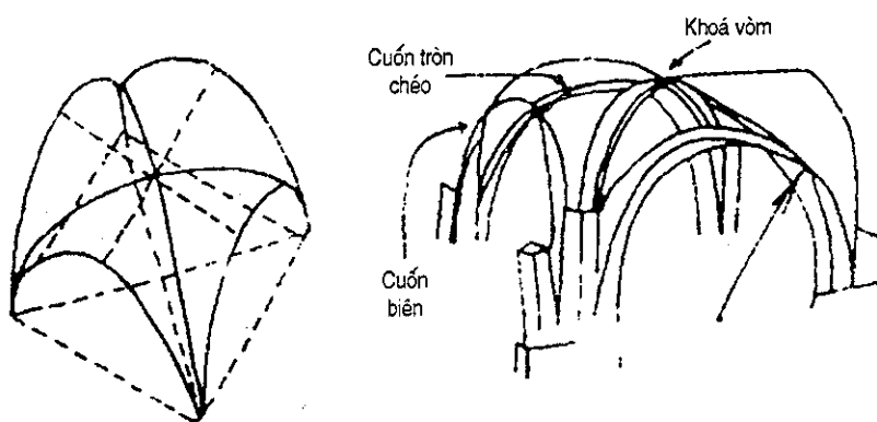
Hệ thống kết cấu vòm Rôman
