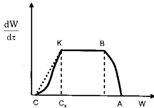
Hình 8.6. Đường cong tốc độ sấy
