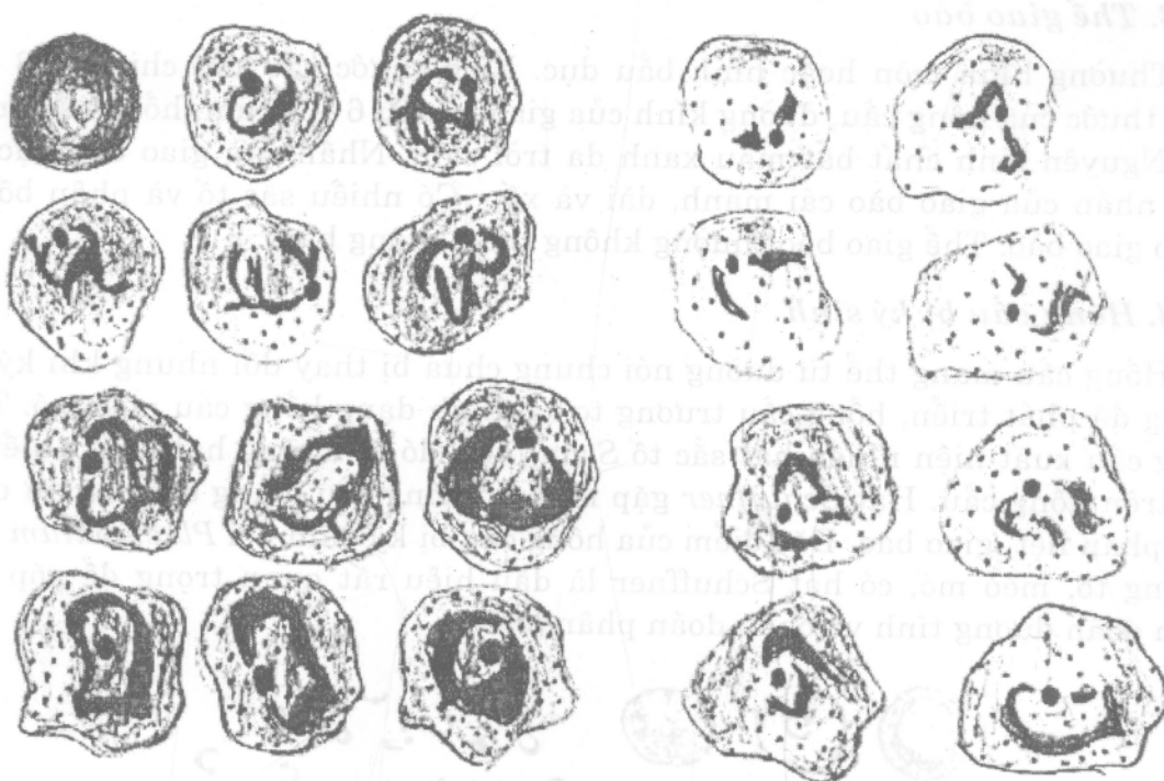
Tư dưỡng
