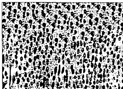
M. audouini
