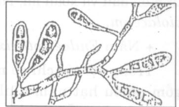
E. floccosum
