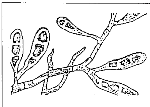
E. floccosum
