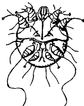
Sarcoptes scabiei
