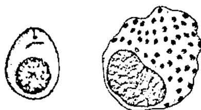
Leishmania
