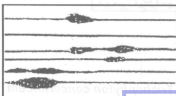
Piedra hortai
