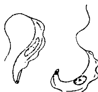
Trypanosoma
