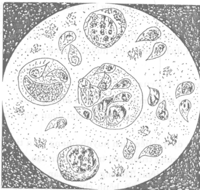
Toxoplasma gondii
