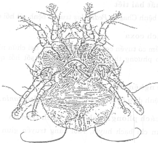
Dermatophagoides pteronyssinus
