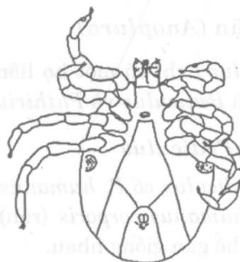
Ixodes crenuatus
