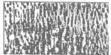
M. audouini
