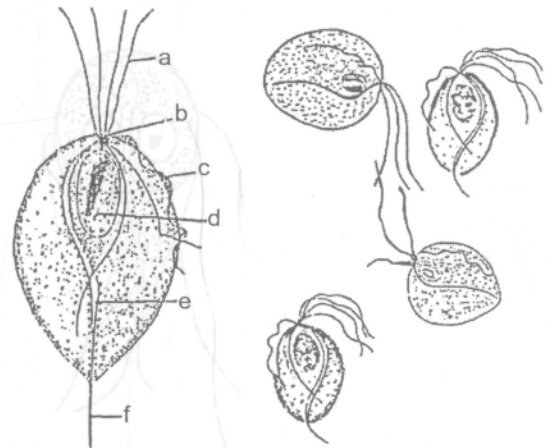
Trichomonas vaginalis
