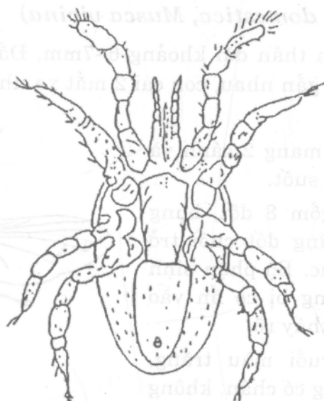
Dermanyssus gallinae
