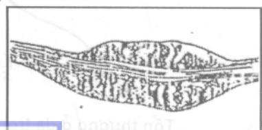
Piedra hortai
