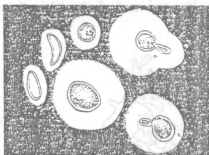
Torulopsis neoformans
