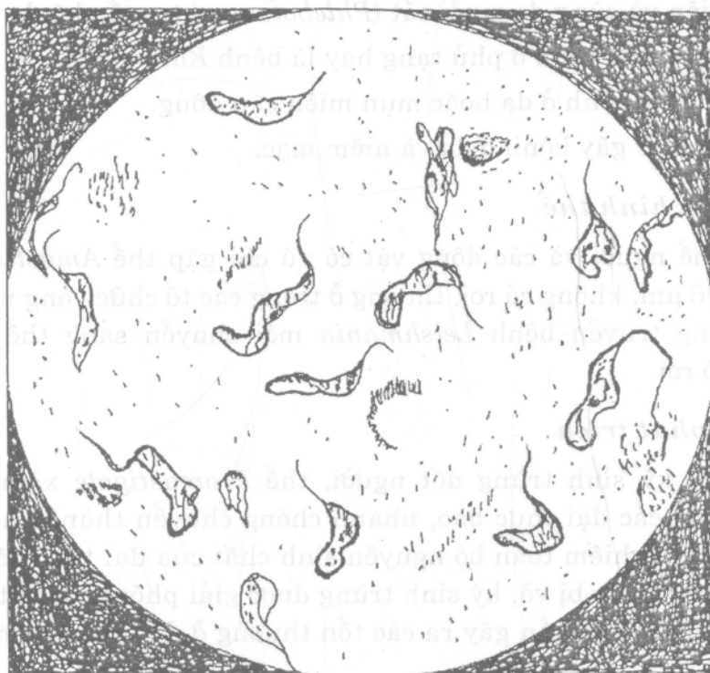
Trypanosoma rhodesiense
