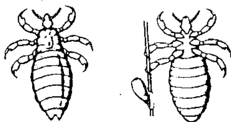
Pediculus capitis
