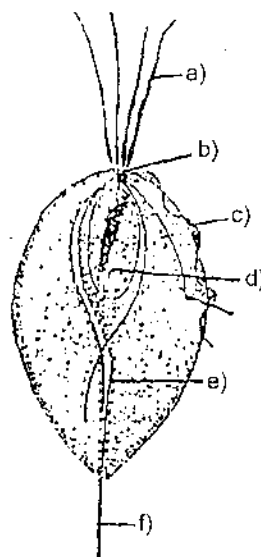
Trichomonas vaginalis
