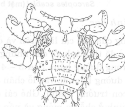
Phthirus pubis
