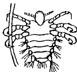
Phthirius pubis
