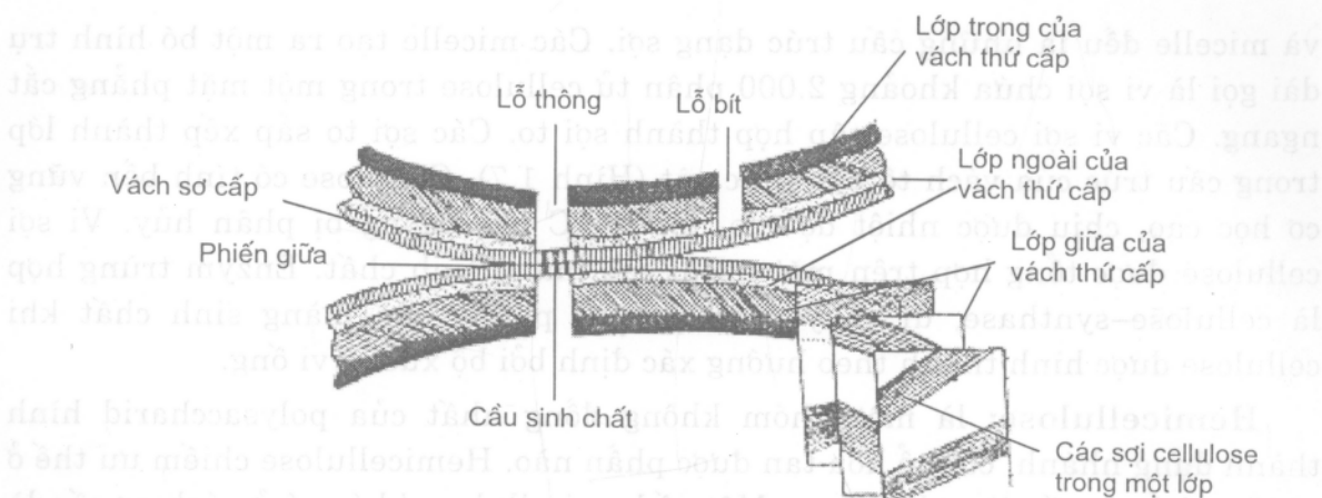
Hình 1.5. Sơ đồ cấu trúc vách tế bào thực vật
