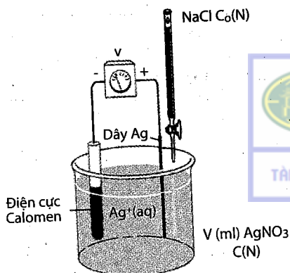
Hình 4.22. Bố trí thí nghiệm chuẩn độ đo thể xác định nồng độ \text{AgNO}_3
