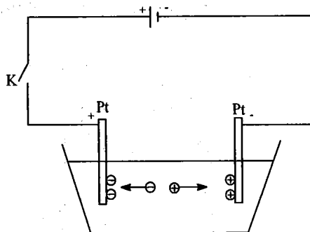
Hình 3.1. Sơ đồ mô tả vật dẫn loại 2
