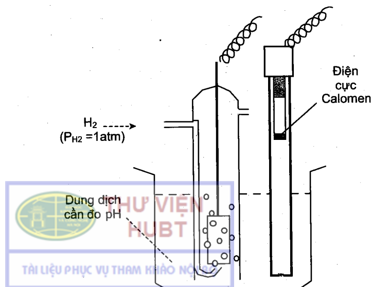
Hình 4.17. Sơ đồ đo pH bằng điện cực hydro
