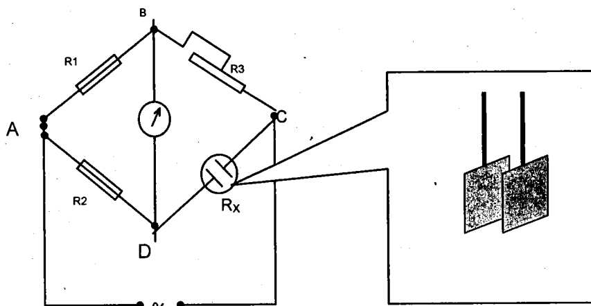
Hình 3.3. Sơ đồ mạch cầu Wheaston
