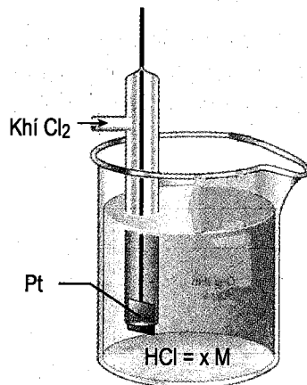
Hình 4.10. Điện cực khí Clo
