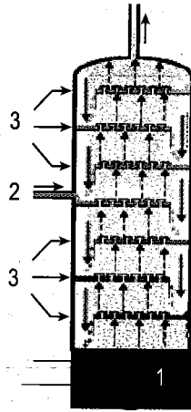
Hình 2.21. Sơ đồ tháp chưng cất tinh luyện
