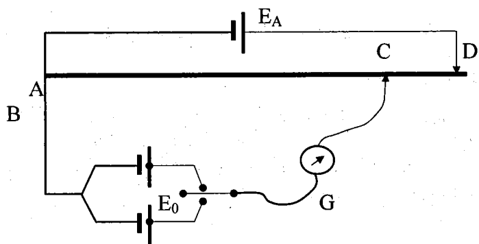
Hình 4.5. Sơ đồ nguyên lý của phương pháp đo sức điện động bằng phương pháp đối xung
