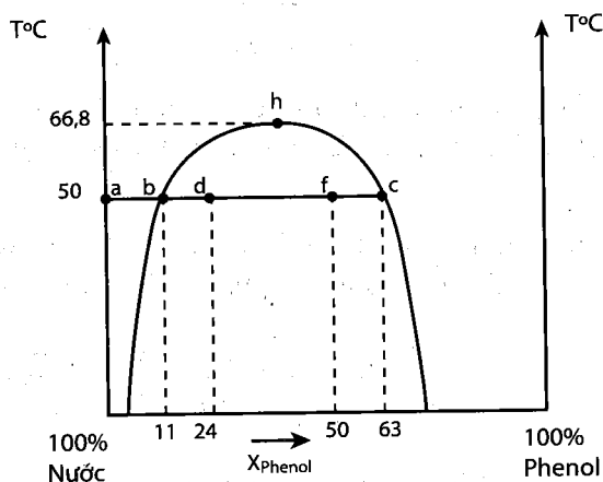
Hình 2.4. Giản đồ pha của hệ phenol - nước
