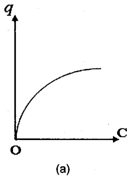
Hình 8.3. Đồ thị biểu diễn phương trình Langmuir dạng đường cong và dạng đường thẳng.
