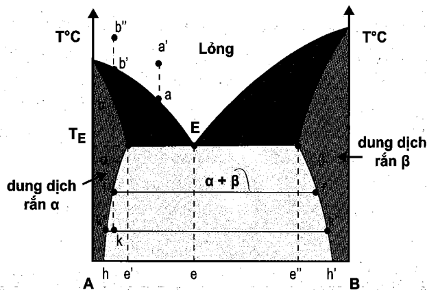
Hình 2.9. Biểu đồ nóng chảy của hệ hai cấu tử hoà tan hạn chế ở pha rắn
