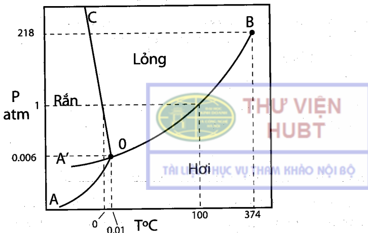
Hình 2.1. Giảm đồ pha của nước ở áp suất trung bình
