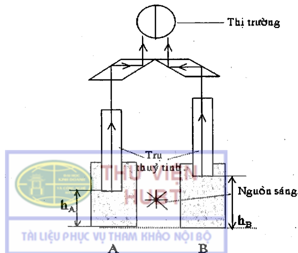
Hình 9.1. Sơ đồ nguyên tắc máy đo độ đục (A - Hệ keo chuẩn, B - Hệ keo cần xác định nồng độ)
