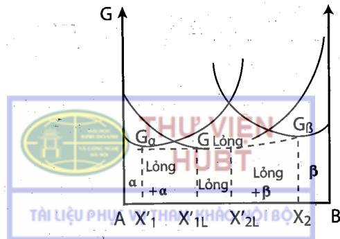
Hình 2.17. Giản đồ thế đẳng áp của hệ hai cấu tử được biểu diễn trên hình 2.15 tại nhiệt độ T_2 > T_E
