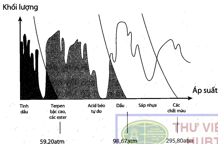
Hình 2.3. Ảnh hưởng của áp suất đến khả năng hòa tan chọn lọc của CO 2 siêu tới hạn ở 60°C đối với một số hợp chất
