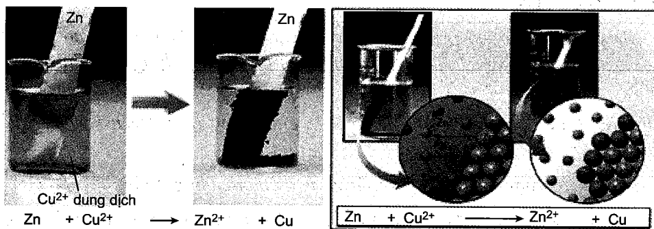
Hình 4.1. Phản ứng oxy hóa Zn trong dung dịch \text{CuSO}_4
