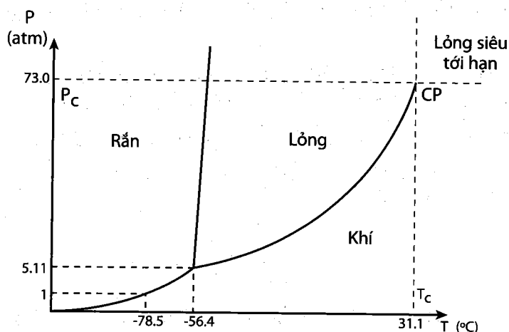
Hình 2.2. Giảm đồ pha của khí CO 2 nén tới trạng thái lỏng siêu tới hạn (CP là điểm tới hạn)
