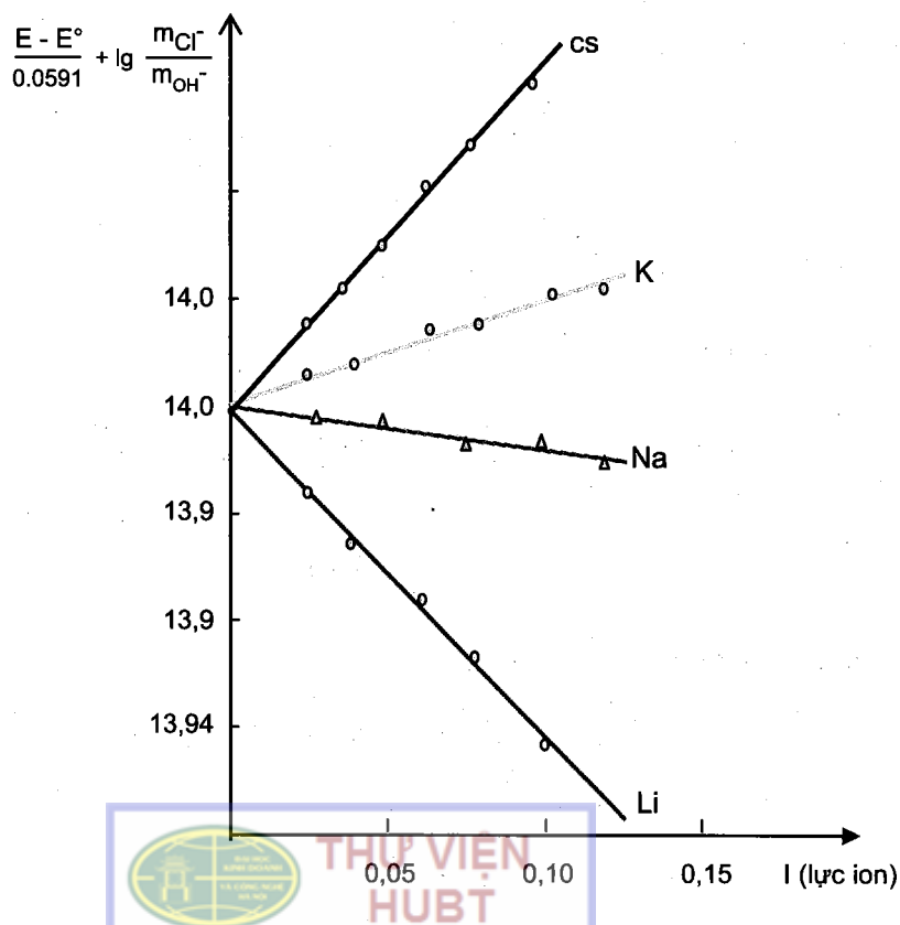
Hình 4.16. Đồ thị biểu diễn sự phụ thuộc của \frac{(E - E^o)}{0,0591} + \lg \frac{m_{Cl^-}}{m_{OH^-}} vào lực ion.
