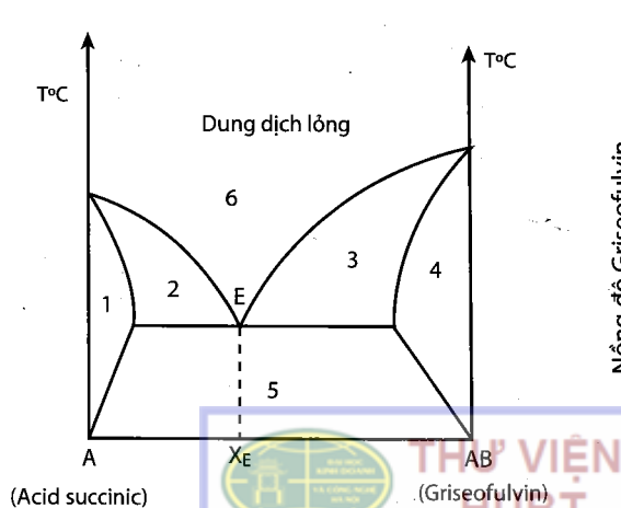
Hình 2.19a. Giản đồ pha hệ griseofulvin - acid succinic
