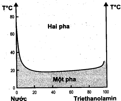
Hình 2.5. Giản đồ pha Hệ triethanolamin – nước
