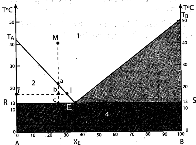
Hình 2.8. Giảm đồ phẳng của hệ thymol - salol
