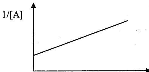
Hình 5.8. Đồ thị sự phụ thuộc của 1/[A] vào thời gian
