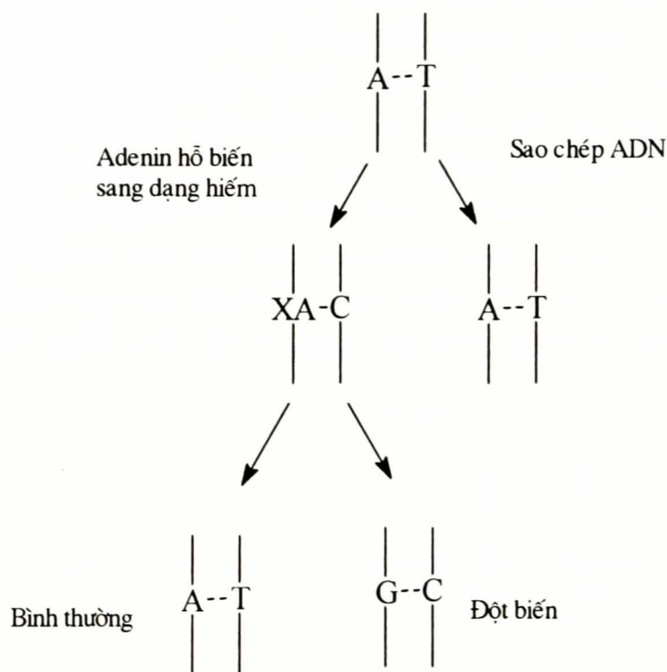
Hình 3.34. Đột biến ngẫu nhiên do adenin hồi biến bất cặp sai trong sao chép
