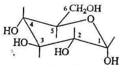
Dạng C1
