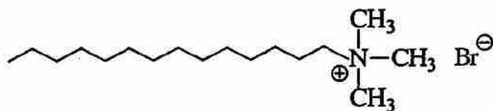
Cetrimonium
