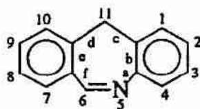
11H-dibenzo [b,e] azepin hay morfantridin
