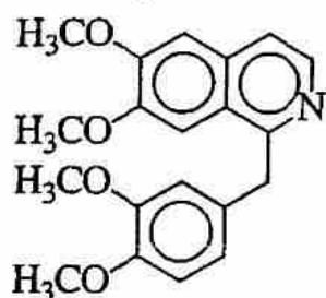
Papaverin
