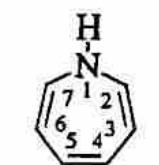
1H-azepin
