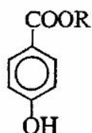
Alkyl p-hydroxy benzoat (chất bảo quản)
