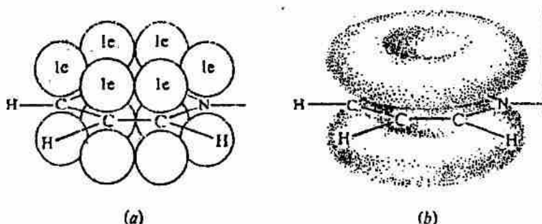
Hình 1. Phân tử pyridin
