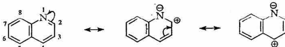
Công thức giới hạn của quinolin
