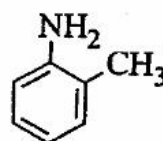
o-Toluidin (o-Tolylamin)
