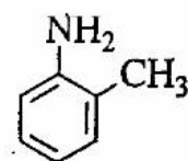
o-Toluidin
