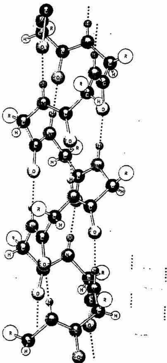
Hình 22.1. Cấu trúc của \alpha -keratin
