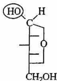
Công thức hình chiếu Fischer
