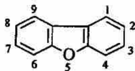
Dibenzofuran
