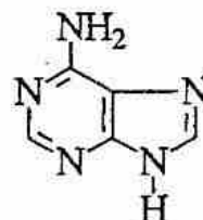
Adenin (6-aminopurin)
