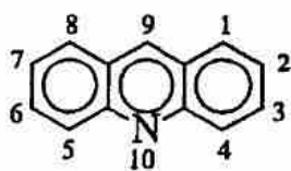
Acridin hay
