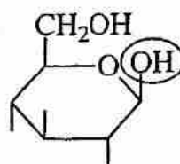
Công thức vòng Haworth
