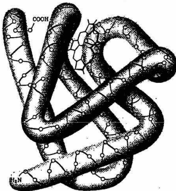
Hình 22.3. Cấu trúc của mioglobin.
