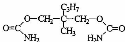
Meprobamat
