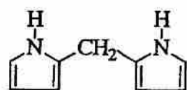
2,2'-Dipyrrolyl methane
