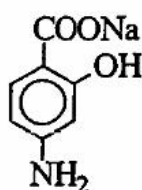
P.A.S sodic (thuốc kháng lao)
