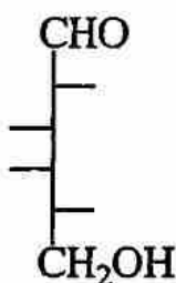
D-galactose
