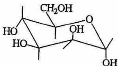
\alpha -D-manopyranose
