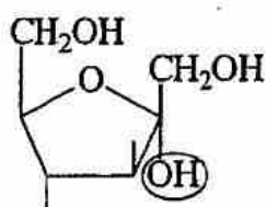
\alpha -D-fructofuranose
