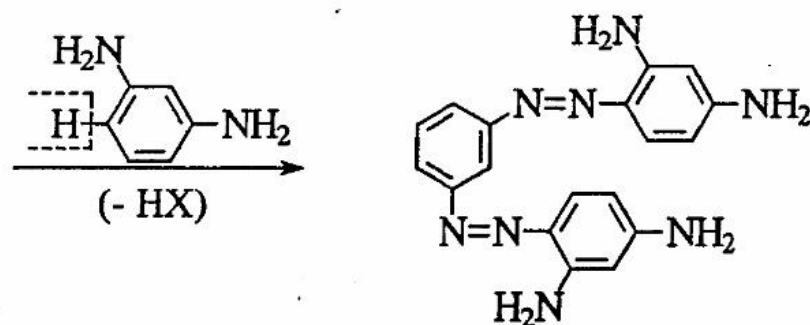
Phẩm màu Bismark
