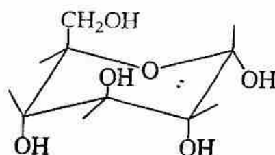
Dạng 1C
