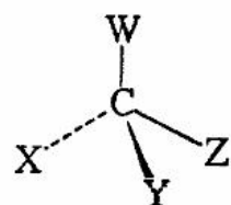
1 alkan chiral
