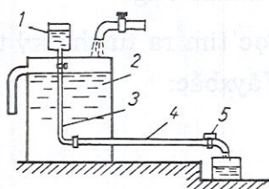
Thiết bị thí nghiệm Rây-nôn
