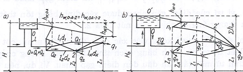
Tính mạng lưới đường ống khép kín
