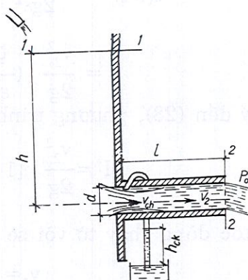
Dòng chất lỏng qua vòi hình hình trụ ngoài
