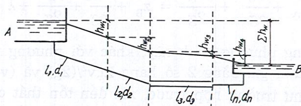
Đường ống nối liên tiếp
