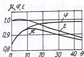
Quan hệ giữa các hệ số của hình nón hội tụ và góc hình nón
