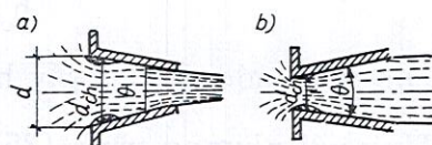
Dòng chảy qua vòi hình nón
