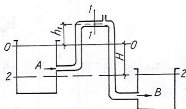
Tính toán ống xiphông
