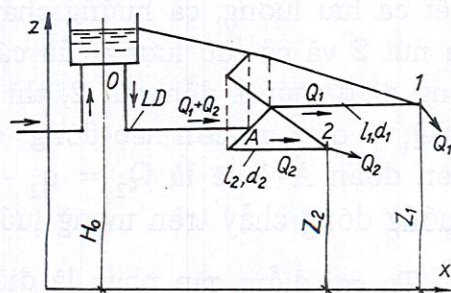
Mạng lưới đường ống hở
