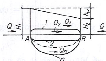
Đường ống nối song song
