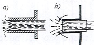
Dòng chảy qua vòi hình trụ gắn trong
