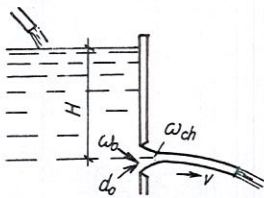
Dòng chất lỏng chảy qua lỗ vào khí quyển
