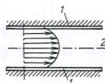
Phân bố vận tốc trong chuyển động rối của chất lỏng trong ống
