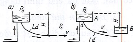
Tính toán đường ống đơn giản
