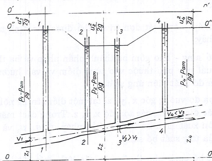
Ý nghĩa hình học của phương trình Becnui đối với dòng chảy của chất lỏng không nhớt
