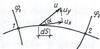
Xác định lưu số vận tốc
