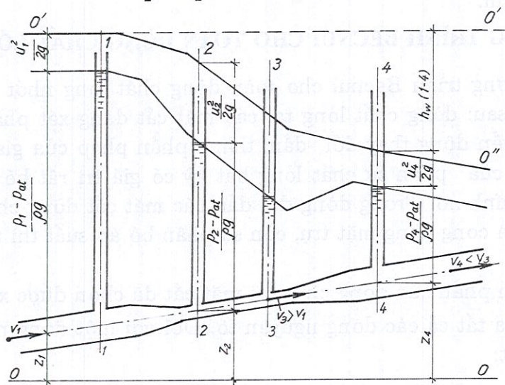
Ý nghĩa hình học của phương trình Becnui cho dòng nguyên tố chất lỏng thực
