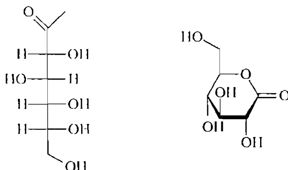
Hình 5.5. Công thức của acid gluconic (A) và glucono-δ-lactone (B)
