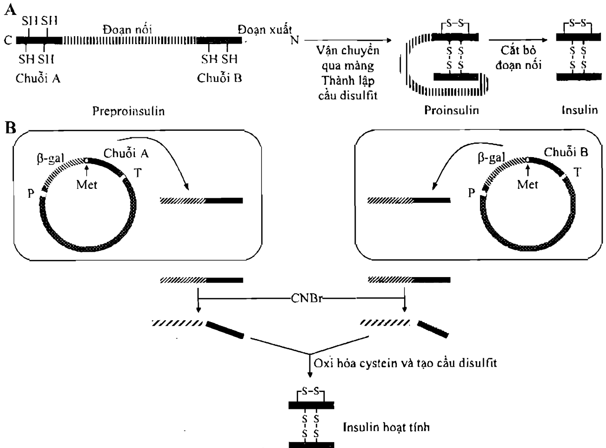
Hình 11.3. Sản xuất insulin tái tổ hợp
