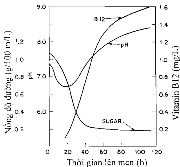
Hình 5.13. Biến đổi động học trong quá trình lên men tủy mè vitamin \text{B}_{12}
